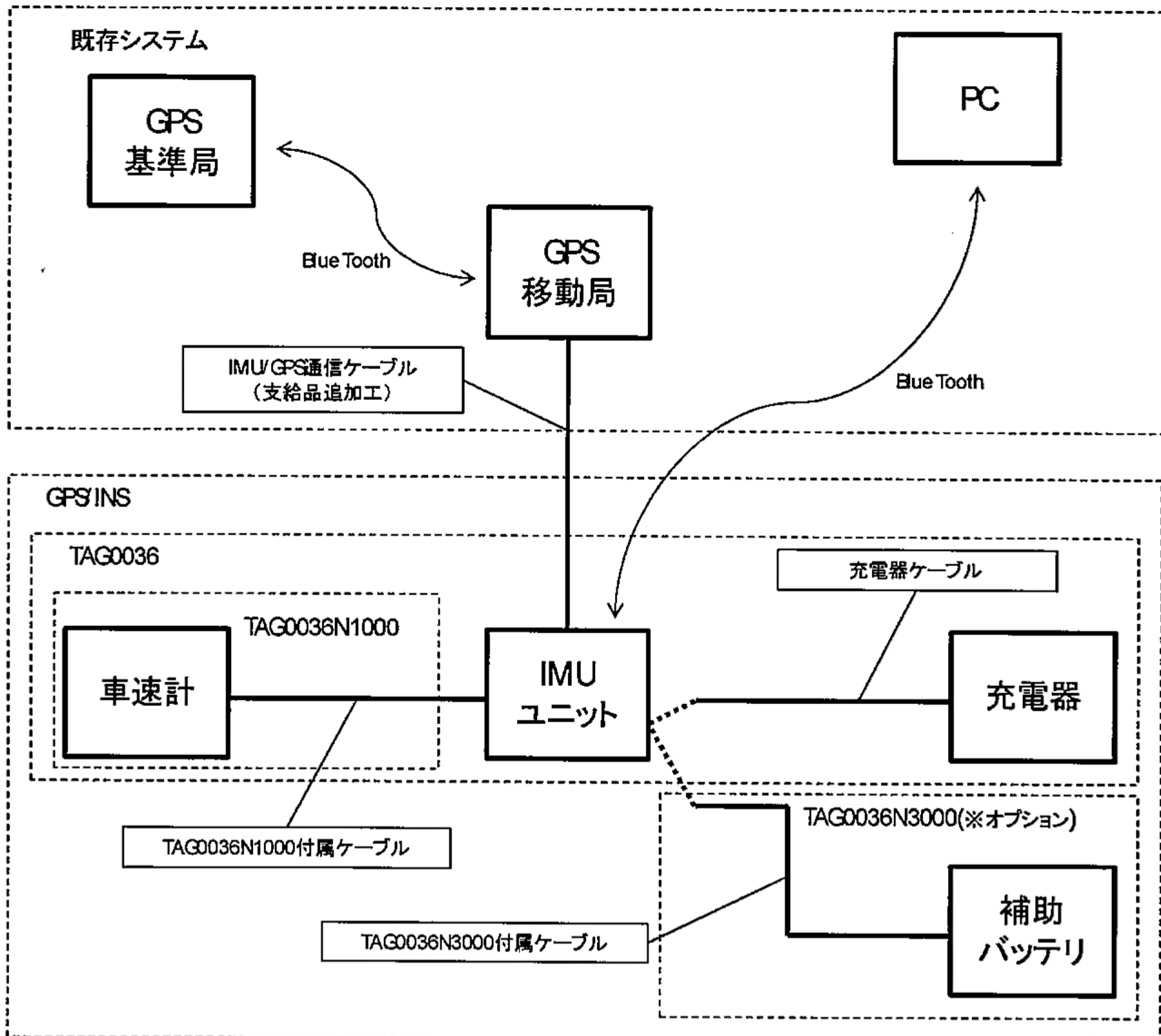
△ 図2-2 機器構成 ブロック図
